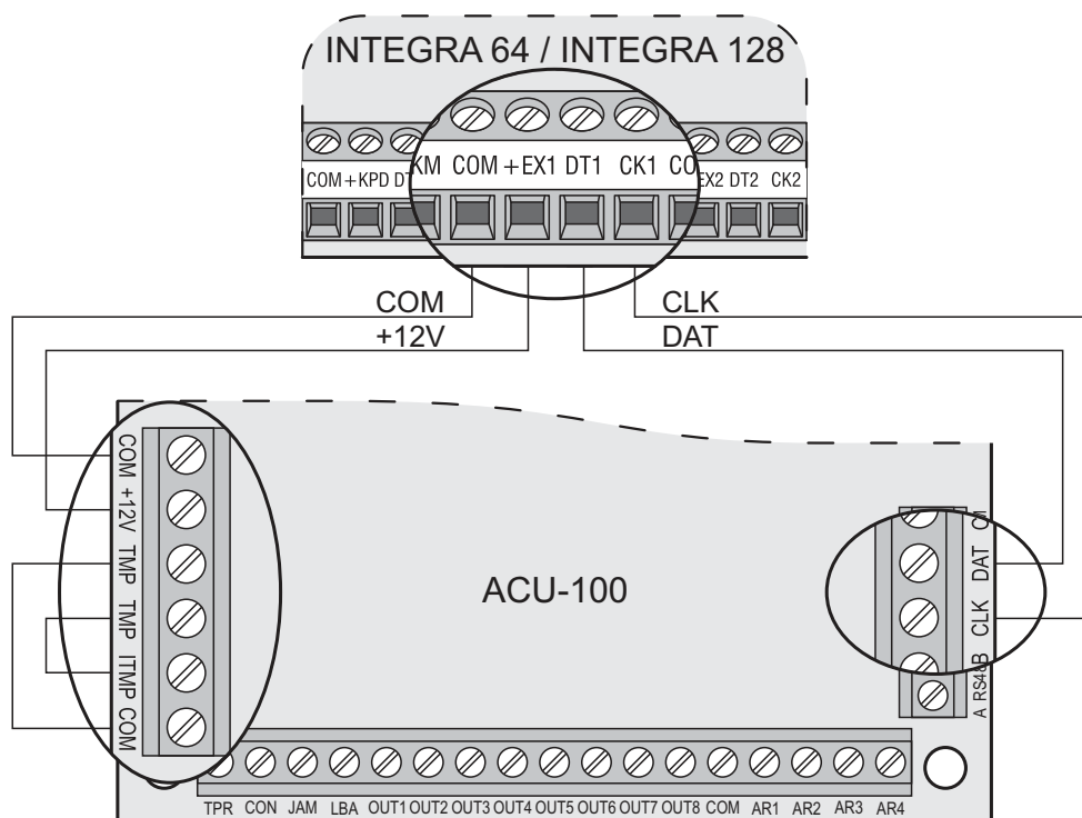
Rys. 8. Przykład podłączenia kontrolera ACU-100 do centrali alarmowej INTEGRA.
