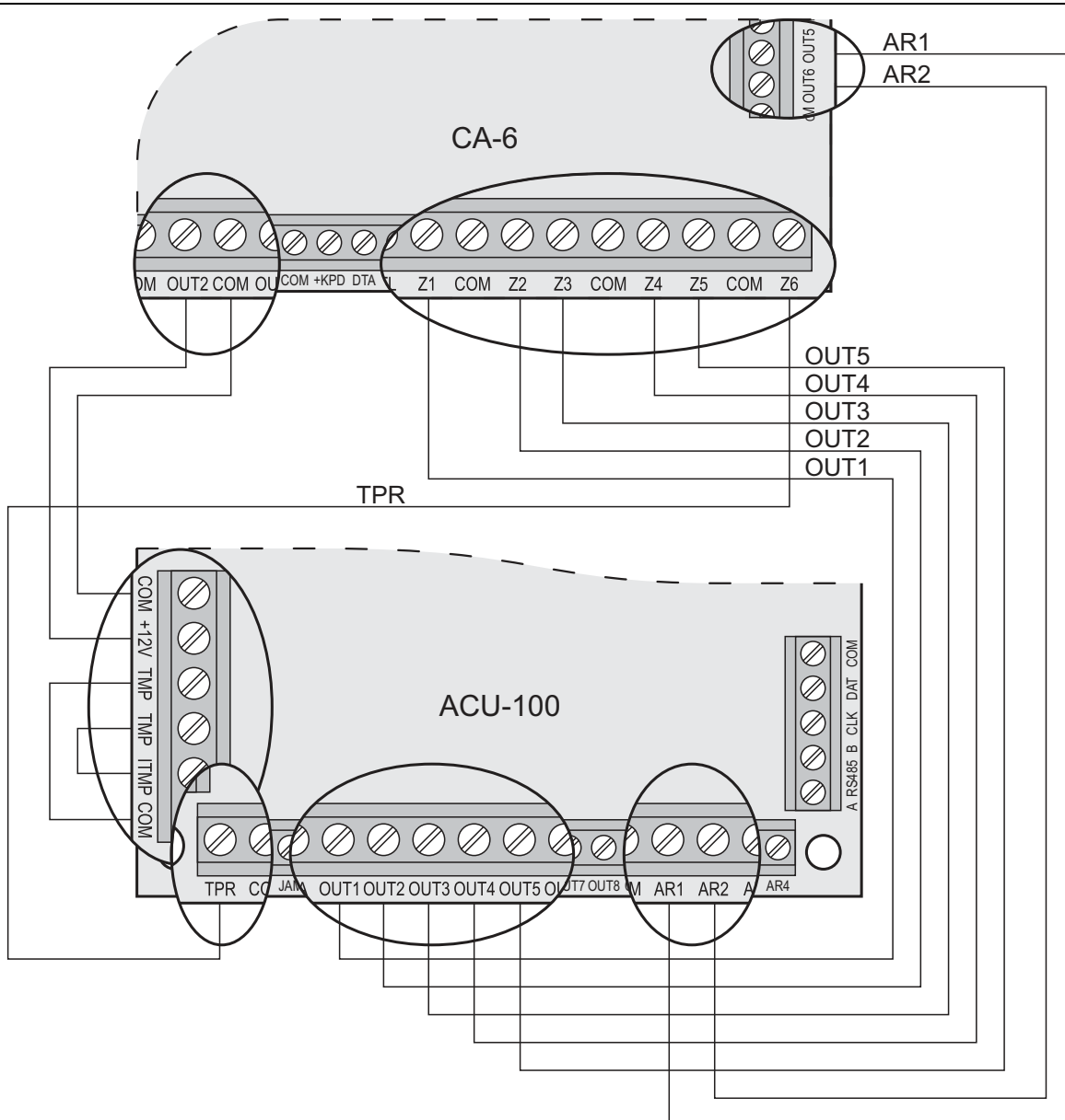
Rys. 14. Przykład podłączenia kontrolera ACU-100 do centrali alarmowej CA-6.
