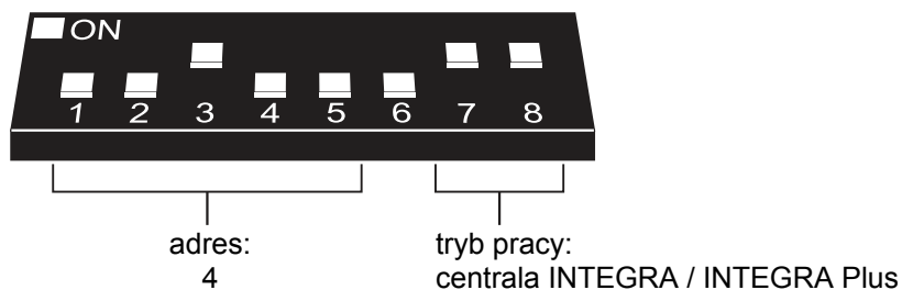
Rys. 7. Przykład ustawienia mikroprzełączników typu DIP-switch.
