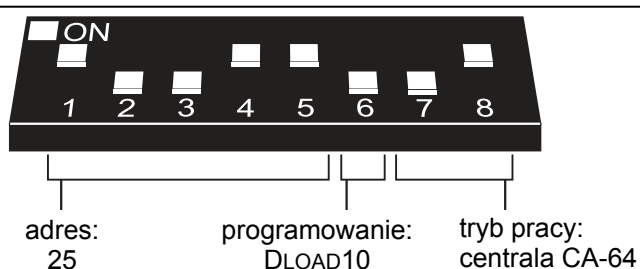
Rys. 9. Przykład ustawienia mikroprzełączników typu DIP-switch.
