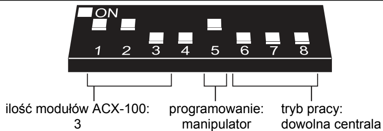
Rys. 13. Przykład ustawienia mikroprzełączników typu DIP-switch.
