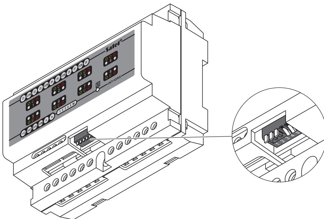
Rys. 1. Ekspander wejść i wyjść INT-IORS. Na powiększeniu pokazano mikroprzełączniki DIP-SWITCH.
